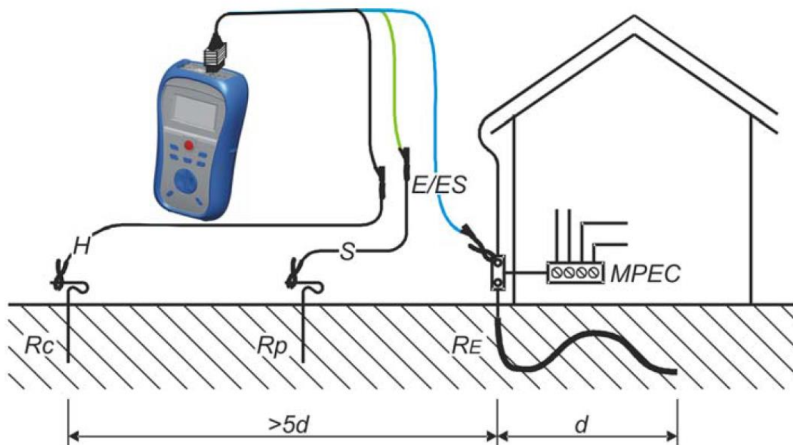
Schéma 4.30: Résistance de terre, mesure de la mise à la terre principale d'une installation
